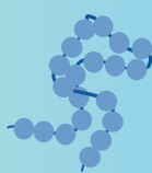
GPCR
