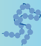
GPCR
